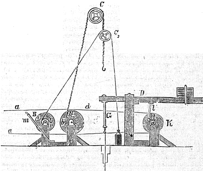
Буровой станокъ Ленца.
