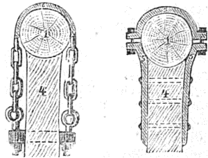
Крѣпленіе В. съ форштевнемъ.
