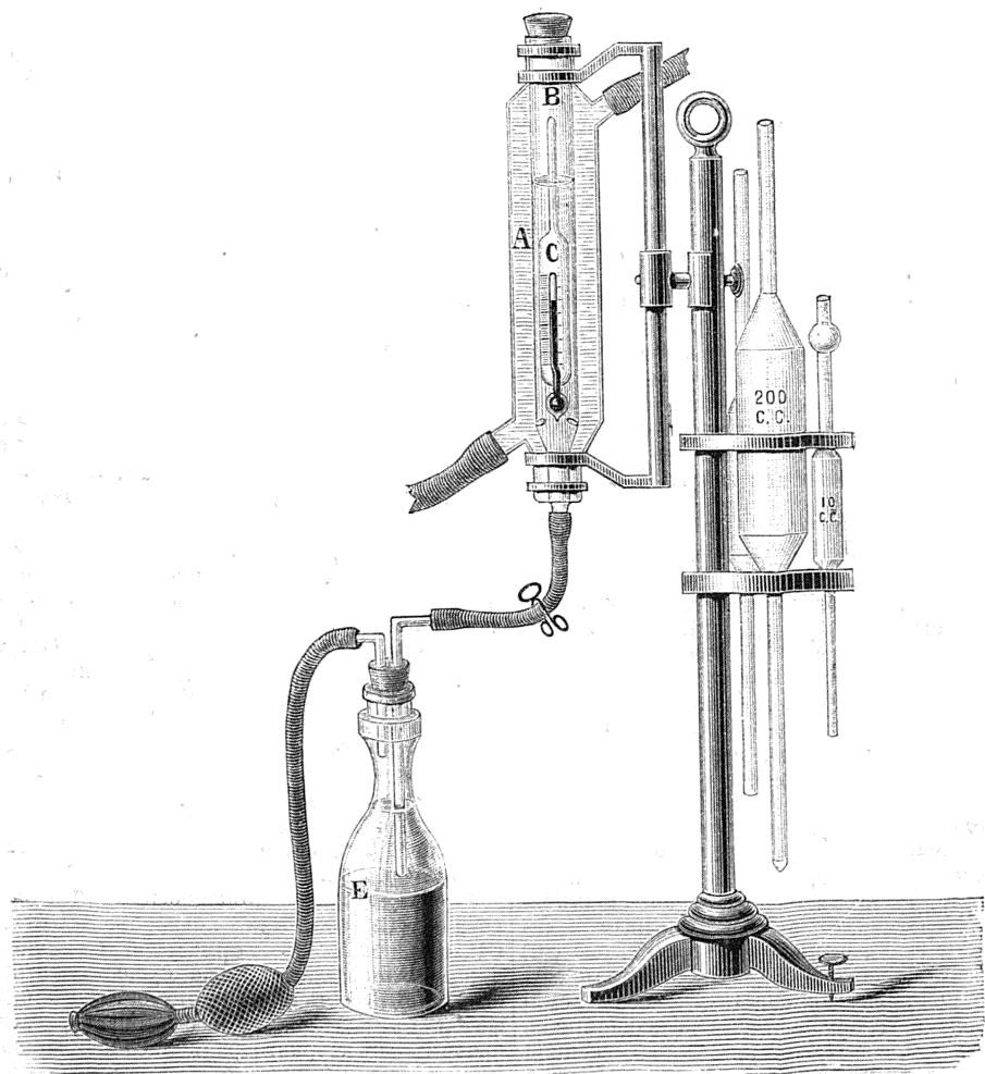
Бутирометръ Сохлета.
